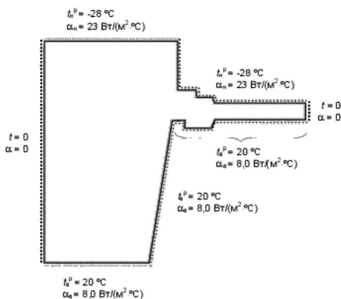
б) Схема заданий граничных условий
