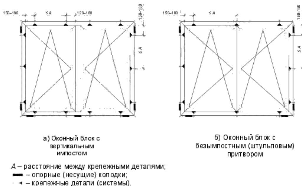
Рисунок Г.2 – Примеры расположения опорных (несущих) колодок и крепежных деталей
