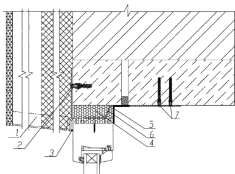
1 – вентилируемый фасад (показан условно); 2 – анкер \Phi 6 \times 60 (шаг крепления – 500 мм); 3 – паропроницаемый герметик; 4 – пенный утеплитель; 5 – паронепроницаемый герметик; 6 – анкерная пластина; 7 – дюбель со стопорным шурупом
