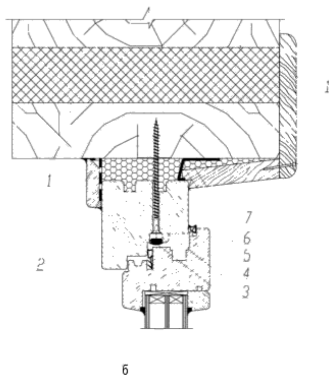
1 — нащельник; 2 — паропроницаемый герметик; 3 — декоративная заглушка; 4 — строительный шуруп; 5 — силиконовый герметик; 6 — пароизоляционный герметик; 7 — пенный утеплитель
